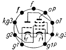
Sockelschaltschema
